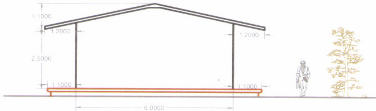
FACHADA LATERAL
