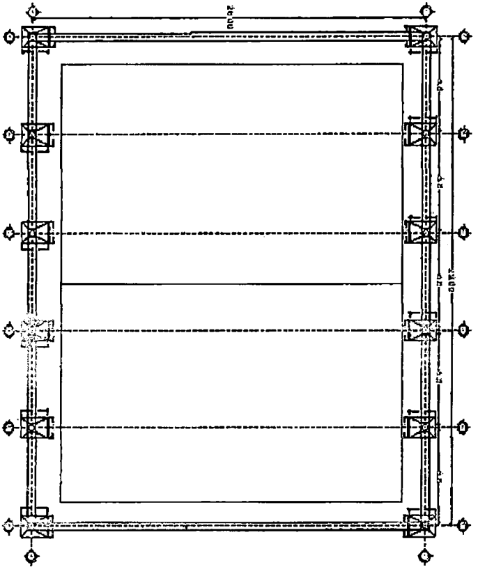
PLANTA DE CIMENTACIÓN
